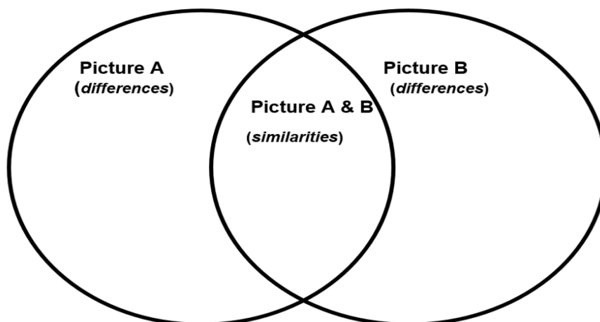
Venn Diagram
